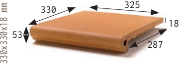
PELDAÑO REDONDEADO 33 ROUNDED STAIR-TREAD 33
