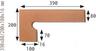
ZANQUÍN REDONDEADO IZDA. ROUNDED STRING LEFT SIDE
