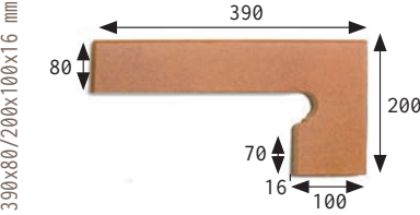
ZANQUÍN REDONDEADO DCHA. ROUNDED STRING RIGHT SIDE
